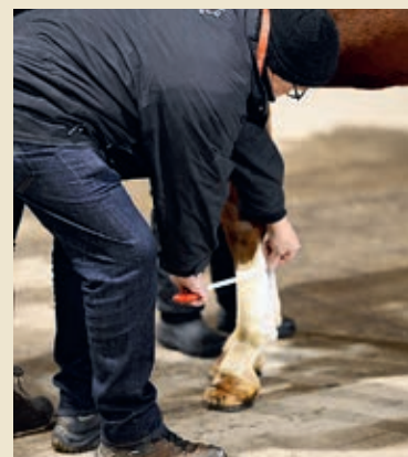
Le secrétaires de concours sont chargés de la toise et de la mesure du tour du canon. / Die Schausekretäre machen die Stockmassmessung sowie Messungen des Röhrbeinumfangs.
