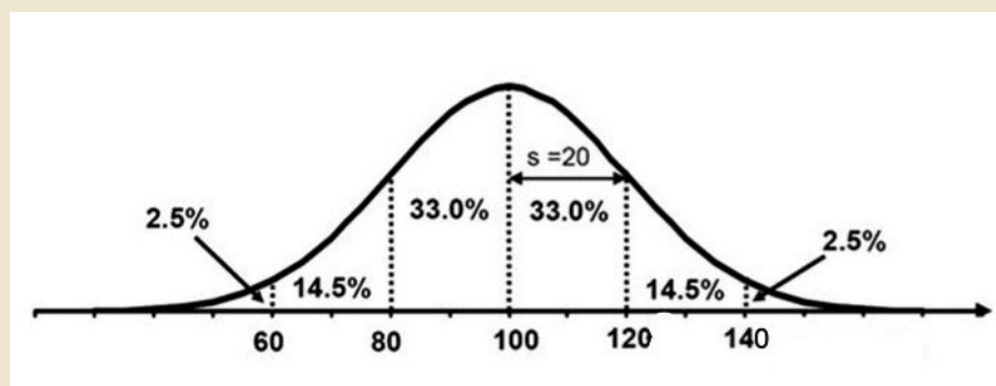
Zuchtwerte: Verteilungskurve.
